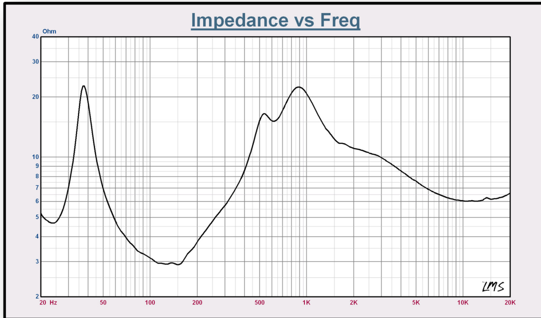
Abbildung 2: Impedanz
