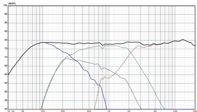
Abbildung 1: Filterung
