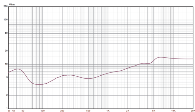
Abbildung 3: Impedanz
