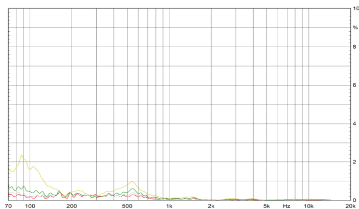
Abbildung 6: Verzerrungen H3 (80dB; 85dB; 90dB; 95dB)
