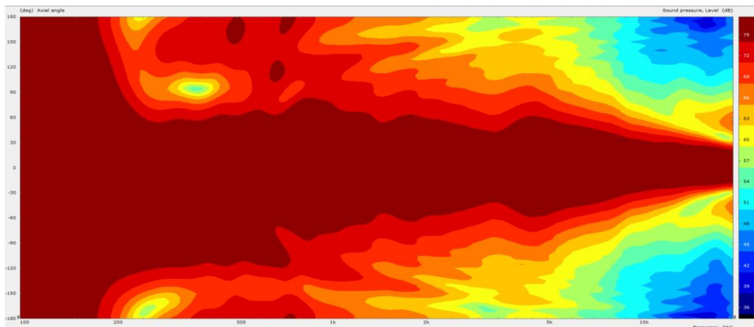
Abbildung 7: Horizontales Abstrahlverhalten (180° - 180°)
