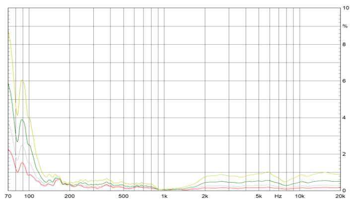
Abbildung 5 : Verzerrungen H2 (80dB; 85dB; 90dB; 95dB)
