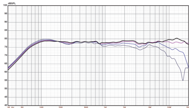
Abbildung 2: Schalldruck 0° - 45° (schwarz 0°)
