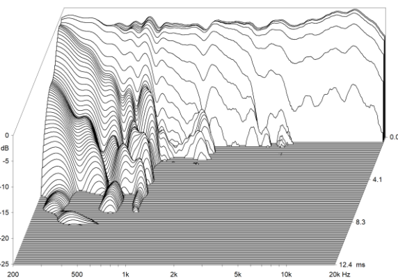
Abbildung 4: CSD
