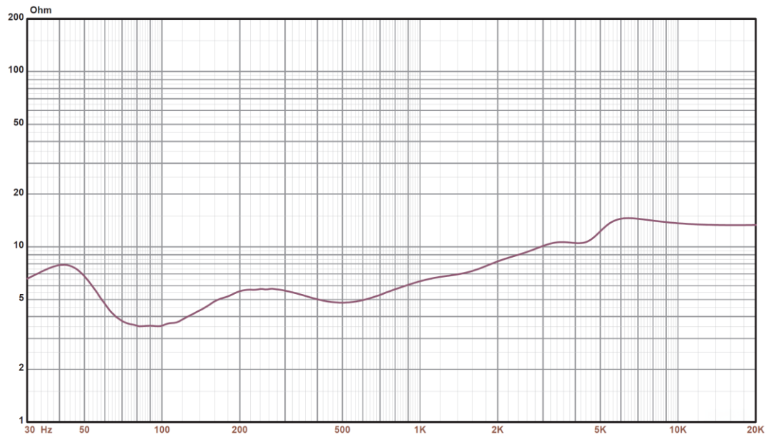
Abbildung 2: Impedanz
