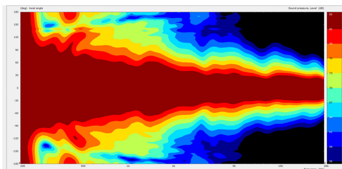
Abbildung 4: Polardiagramm -180° -180° horizontal
