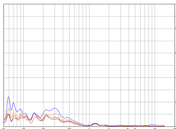
Abbildung 6: Verzerrungen H3 80dB – 105dB
