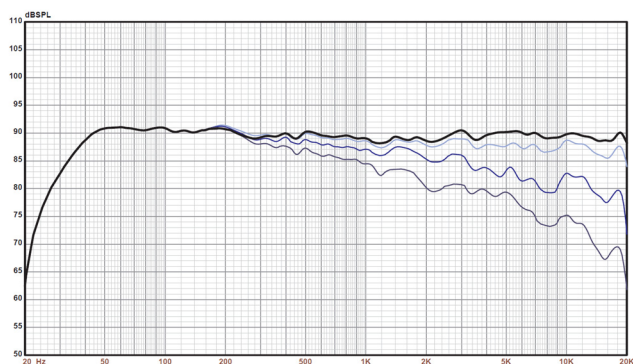
Abbildung 1: SPL 0° - 45° horizontal
