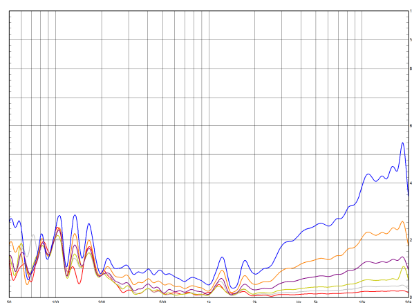
Abbildung 5 : Verzerrungen H2 80dB -105dB
