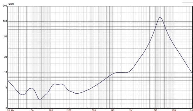
Abbildung 2: Impedanz
