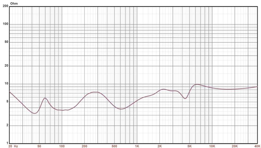
Abbildung 2: Impedanz
