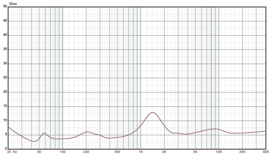
Abbildung 2: Impedanz
