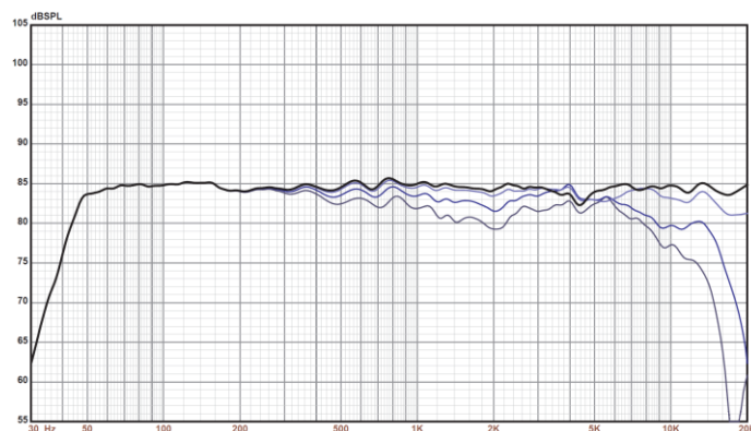
Abbildung 2: Schalldruck 0° -45°
