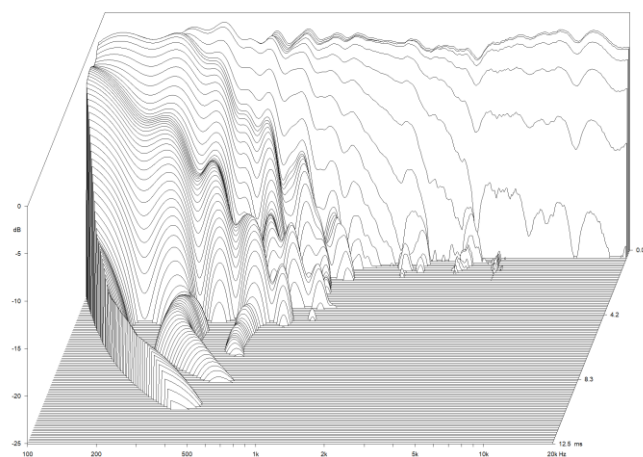
Abbildung 4: CSD
