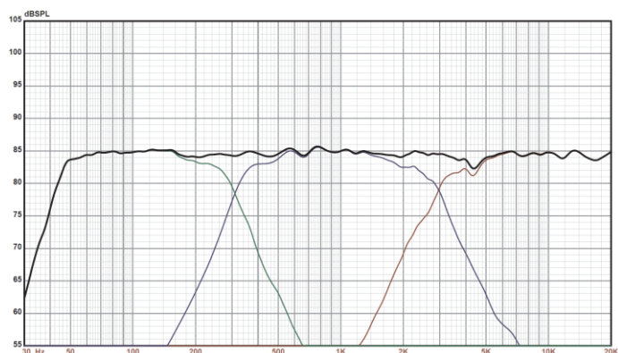
Abbildung 1: Filterung
