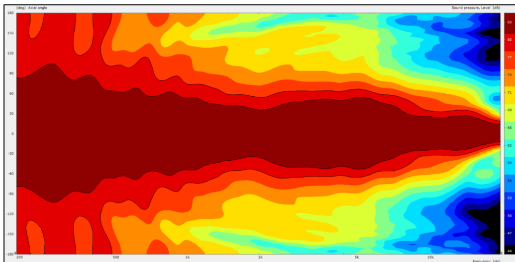
Abbildung 7: Horizontales Abstrahlverhalten (180° - 180°)
