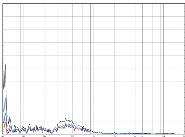
Abbildung 6: Verzerrungen H3 (85dB; 90dB; 95dB, 100dB)
