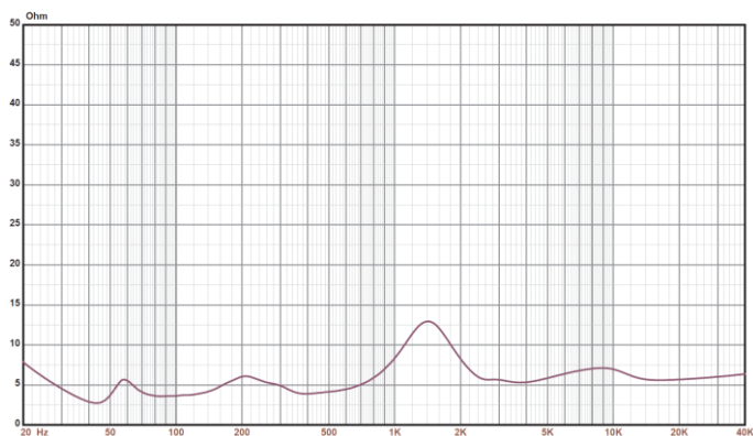
Abbildung 3: Impedanz
