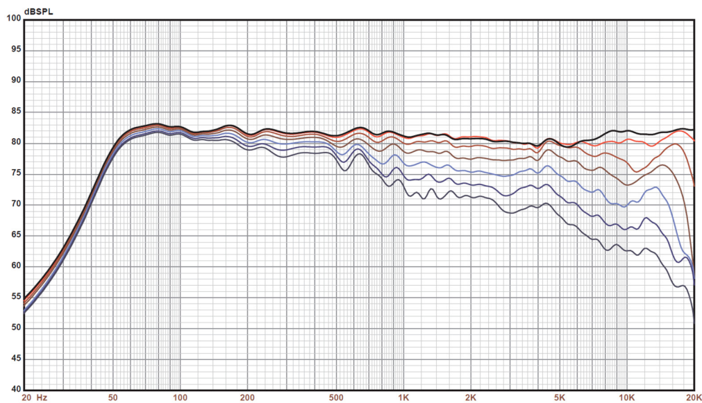
Abbildung 1: Schalldruckverlauf von 0° bis 90°
