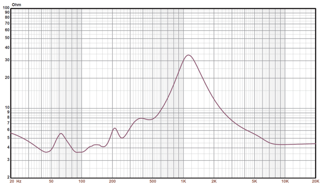
Abbildung 2: Impedanz
