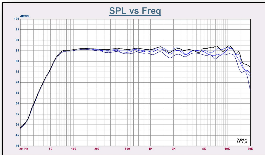
Abbildung 1: Schalldruckverlauf von 0° bis 45°
