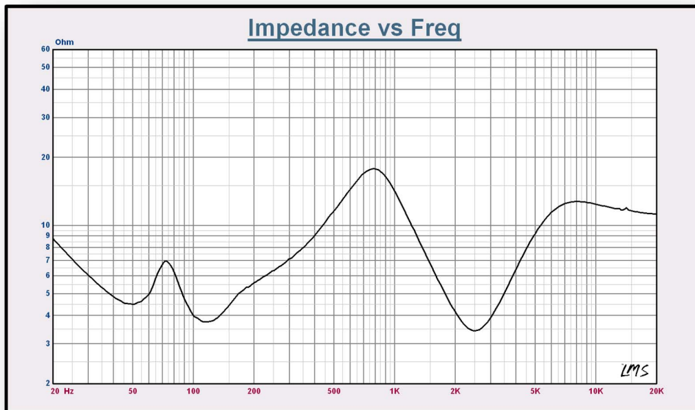
Abbildung 2: Impedanz
