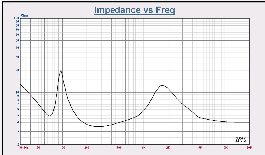
Abbildung 2: Impedanz
